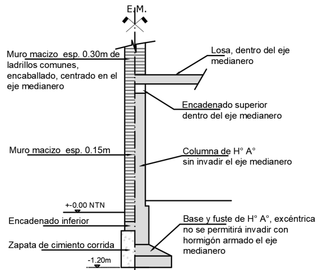
CORTE 2-2
