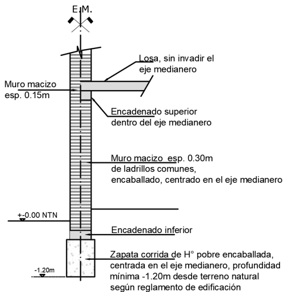
CORTE 1-1
